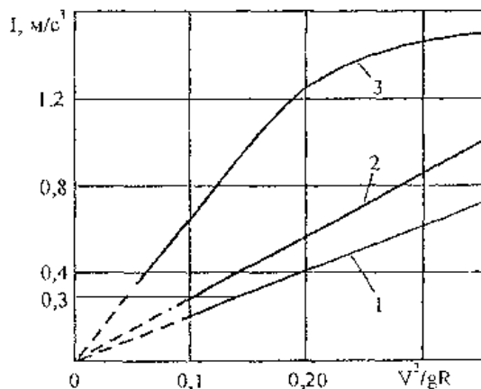
Рис. 4.2. График для определения расчетного нарастания центробежного ускорения
