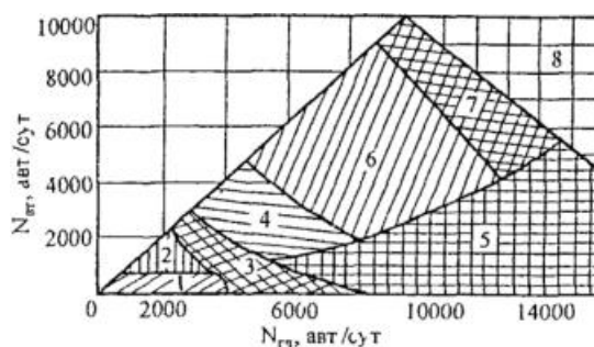
Рис. 8.1. Номограмма для выбора типа планировочных решений пересечений:
