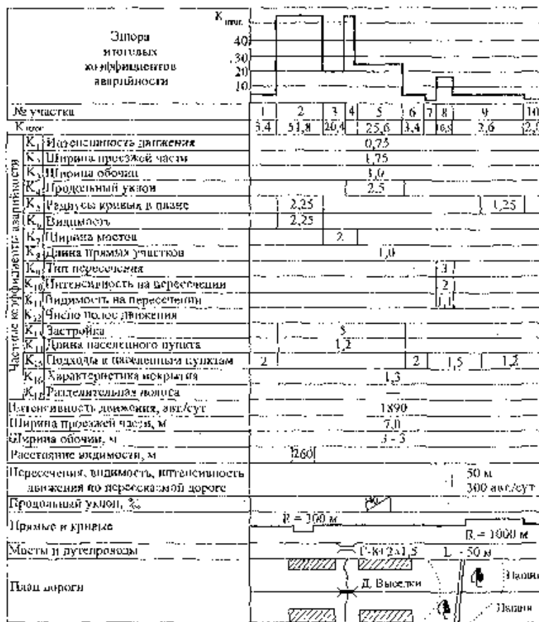
Рис. 1.2. Пример графика итогового коэффициента аварийности
