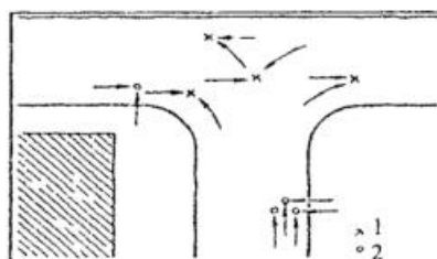
Рис. 8.9. План пересечения с нанесенными на него схемами дорожно-транспортных происшествий:
